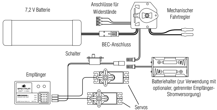
Bild A – Verbindung zwischen BEC und Empfänger mit mechanischem Fahrtregler. Die NiMh-Akkus und der Fahrtregler sind im Lieferumfang der RC-Anlage nicht inbegriffen.
